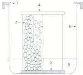
Sezione longitudinale fumigatore
